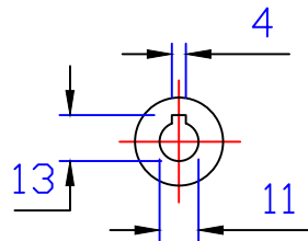
入力孔 Input hole
